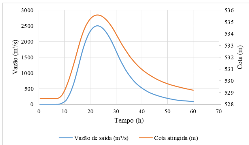
QUADRO 1.13 – BARRAGEM CAMALAUÍ: HIDROGRAMAS DAS VAZÕES DE PROJETO AFLUENTES (QE) E EFLUENTES (QS) E COTAS ATINGIDAS PARA TR=10.000 ANOS
