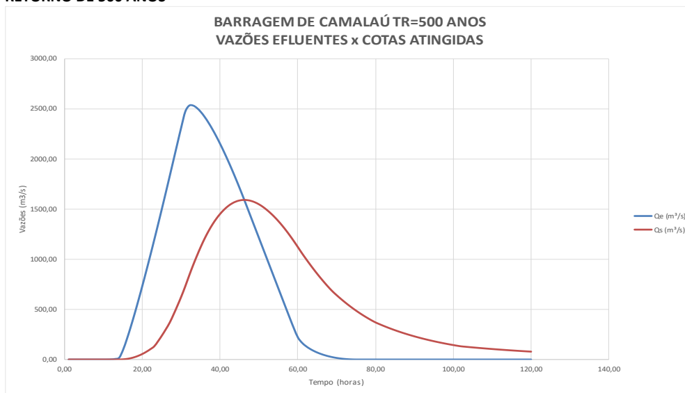
FIGURA 1.8 – BARRAGEM CAMALAUÁ: HIDROGRAMAS EFLUENTES E COTAS ATINGIDAS PARA TEMPO DE RETORNO DE 500 ANOS
