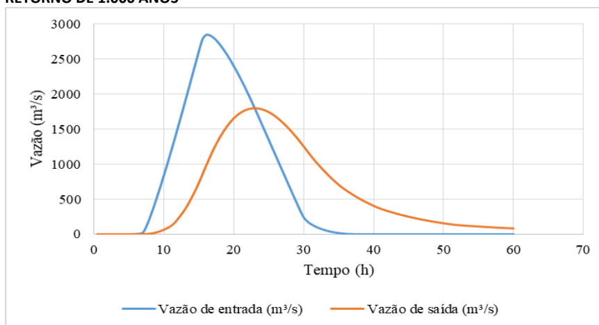
FIGURA 1.9 – BARRAGEM CAMALAUÍ: HIDROGRAMAS DE ENTRADA E SAÍDA PARA TEMPO DE RETORNO DE 1.000 ANOS
