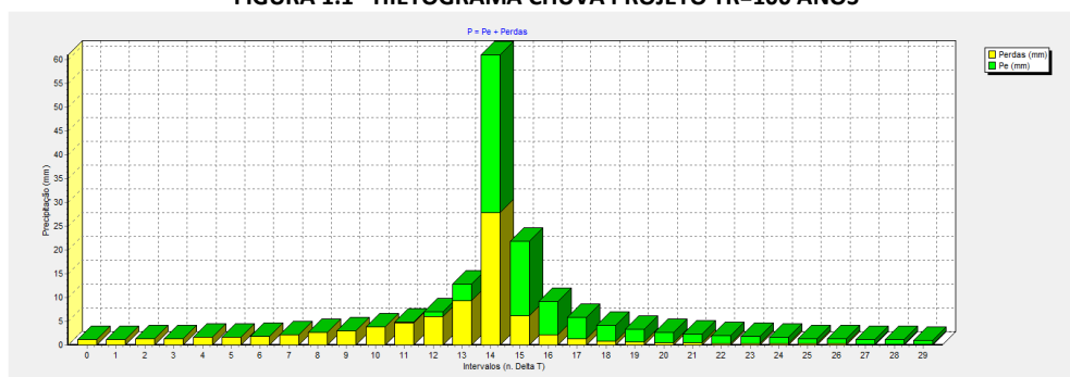
FIGURA 1.1 - HIETOGRAMA CHUVA PROJETO TR=100 ANOS
