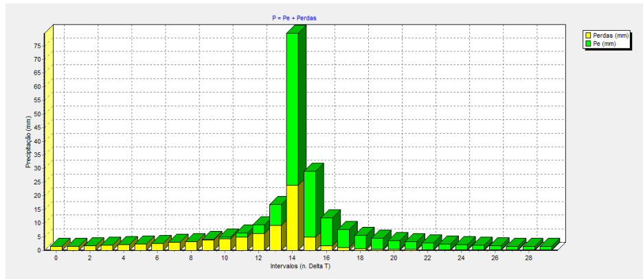
FIGURA 1.4 - HIETOGRAMA CHUVA PROJETO TR=10.000 ANOS
