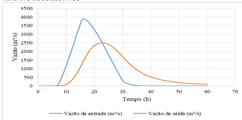
FIGURA 1.12 – BARRAGEM CAMALAUÍ: HIDROGRAMAS EFLUENTES E COTAS ATINGIDAS PARA TEMPO DE RETORNO DE 10.000 ANOS
