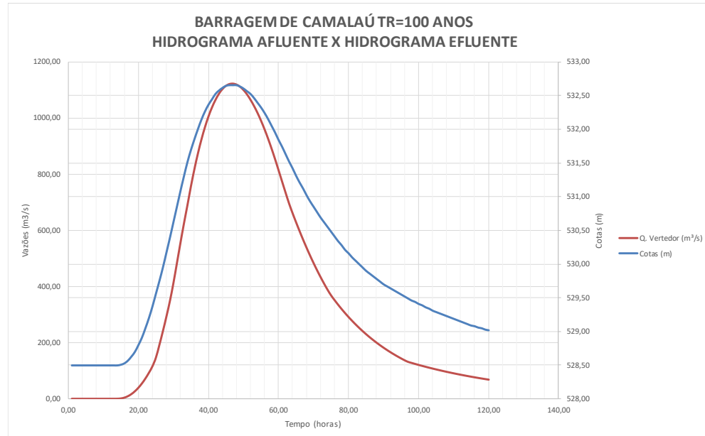
QUADRO 1.10 – BARRAGEM CAMALAÚ: HIDROGRAMAS DAS VAZÕES DE PROJETO AFLUENTES (QE) E EFLUENTES (QS) E COTAS ATINGIDAS PARA TR=100 ANOS
